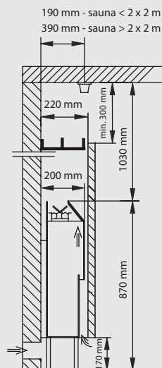
Montagebeispiel Bi-O Mat U
