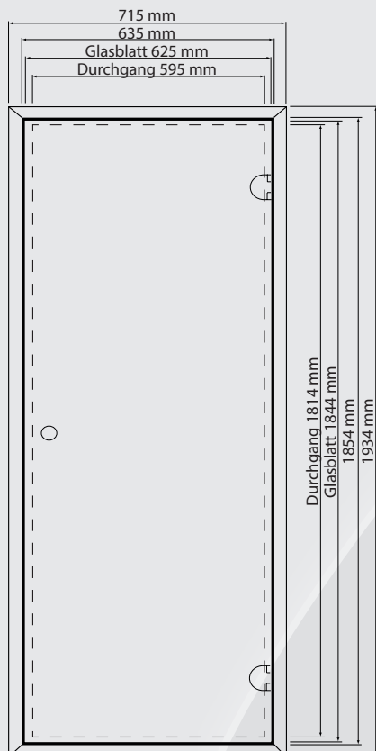
Maße der Saunatüren Basic und Premium
