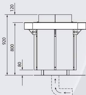
Zuluft über Zuluftkanal ggf. mit Lüfter Air supply via channel, fan may be required
