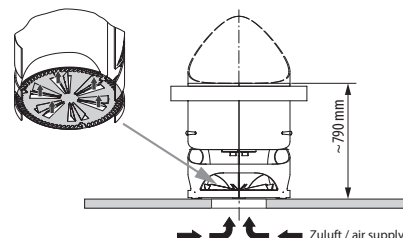
Installation in der Kabinenmitte oder vor einer Glaswand – Zuluft von unten. Mindestmaß der be- und Entlüftung 50 x 10 cm (ca. 500 cm 2 ) / Ø 30 cm
