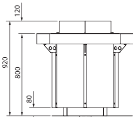
Zuluft über Zuluftkanal ggf. mit Lüfter Air supply via channel, fan may be required
