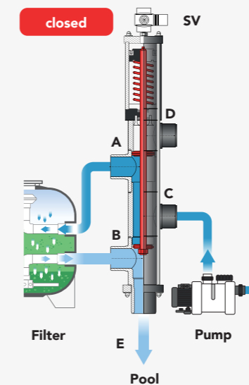
SV Elektromagnetisch ventiel A Filteraansluiting (inlaat) B Filteraansluiting (uitlaat) C Aansluiting op filtratiepomp
