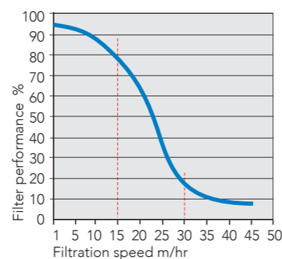
Bij halvering van de filtratiesnelheid van 30 tot 15 m/u verbetert het rendement met factor 4.
