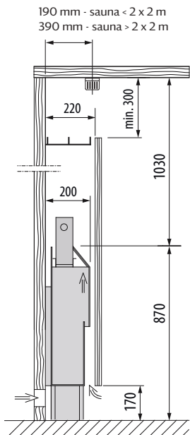
Abb. Verdampfer linksseitig
