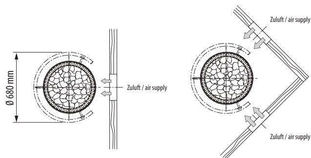
Ofenberührungsschutz optional
