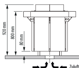
Ofenberührungsschutz optional
