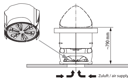
Ofenberührungsschutz optional
